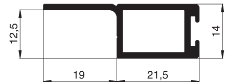
10 34 28 Montagerahmenprofil
