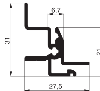
10 33 22 Adapterprofil
