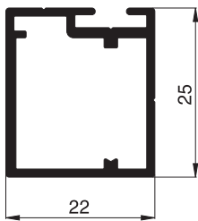
10 35 31 Montagerahmenprofil
