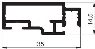
10 35 02 Drehrahmenprofil
