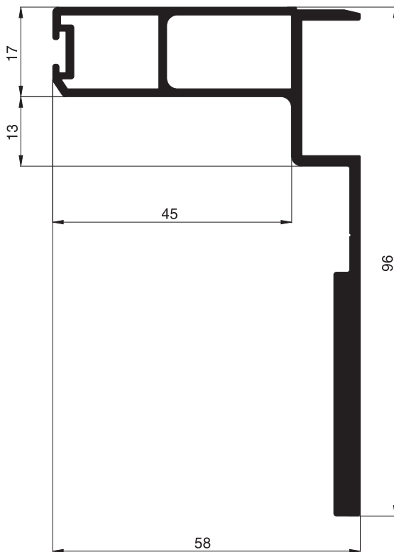
10 32 18 Statikprofil
