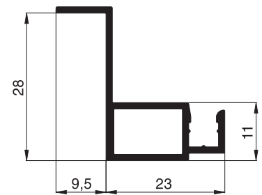
10 23 07 Spannrahmenprofil
