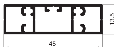
10 46 12 unteres Montagerahmenprofil
