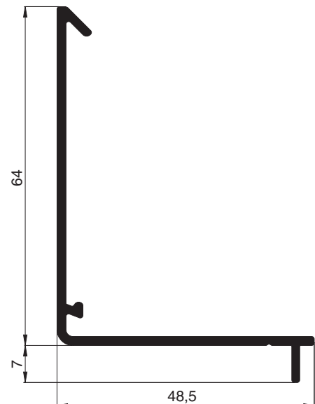
10 43 02 Kastenblende
