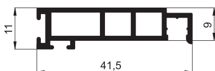
10 24 56 Spannrahmenprofil
