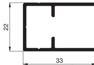
10 45 04 Rahmenprofil
