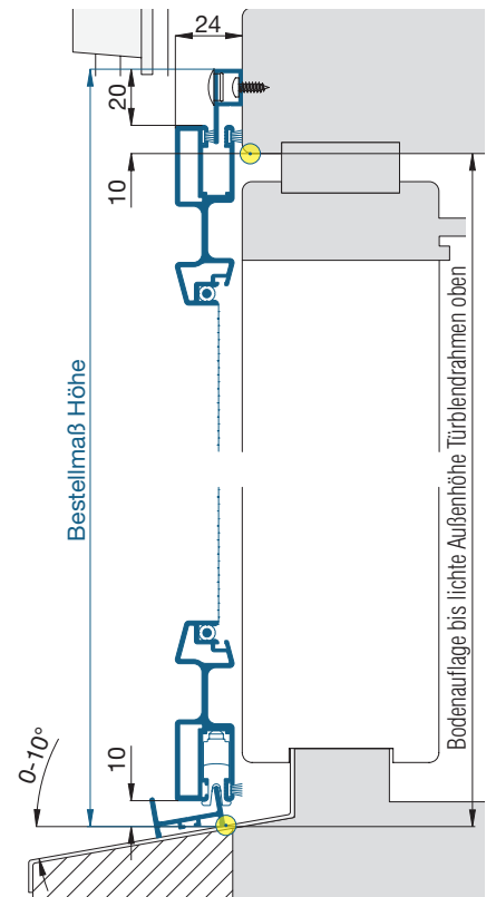
Vertikalschnitt, M 1:3
