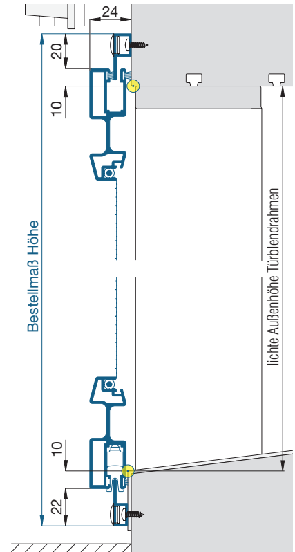
Vertikalschnitt, M 1:3
