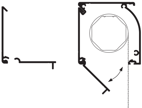
2-teilige Kastenblende
