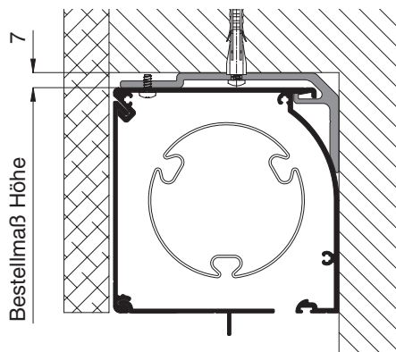
Deckenmontage
