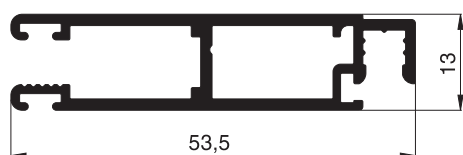
10 48 02 Schiebeflügelprofil
