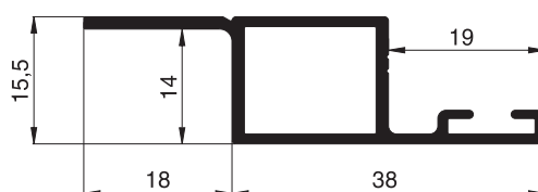
10 35 24 Montagerahmenprofil
