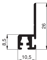
10 35 61 h-Profil
