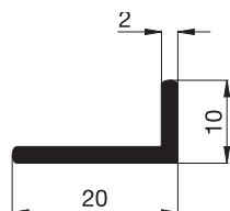
10 90 35 Winkelprofil 20/10/2
