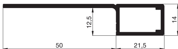
10 34 29 Montagerahmenprofil
