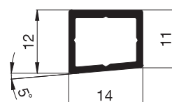
10 34 32 (nur in E1 lieferbar) Schwellenprofil 12 mm
