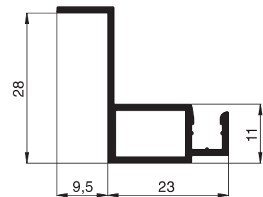
10 23 07 Spannrahmenprofil
