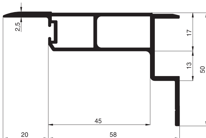
10 32 14 Lichtschachtabdeckungsprofil
