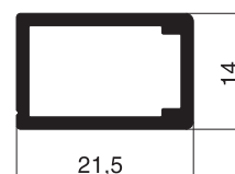
10 34 22 Montagerahmenprofil
