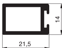
10 34 23 Montagerahmenprofil
