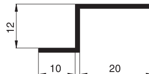
10 26 07 Z-Schiene
