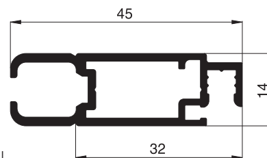
10 34 07 Pendeltürprofil
