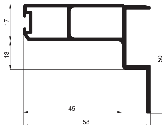
10 32 16 Lichtschachtabdeckungsprofil
