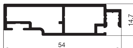
10 35 52 Drehrahmenprofil
