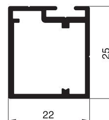
10 35 31 Montagerahmenprofil
