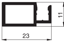
10 23 02 Spannrahmenprofil
