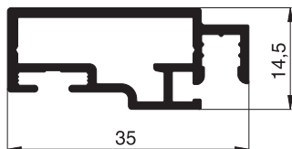
10 35 02 Drehrahmenprofil
