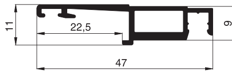
10 22 04 Spannrahmenprofil
