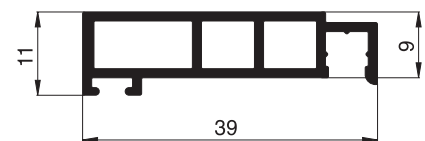
10 24 52 Spannrahmenprofil
