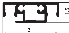
10 35 11 Sprossenprofil
