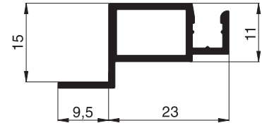
10 23 04 Spannrahmenprofil
