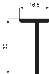
10 45 40 (nur in G5 und S1 lieferbar) Montageprofil
