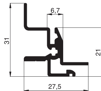
10 33 22 Adapterprofil
