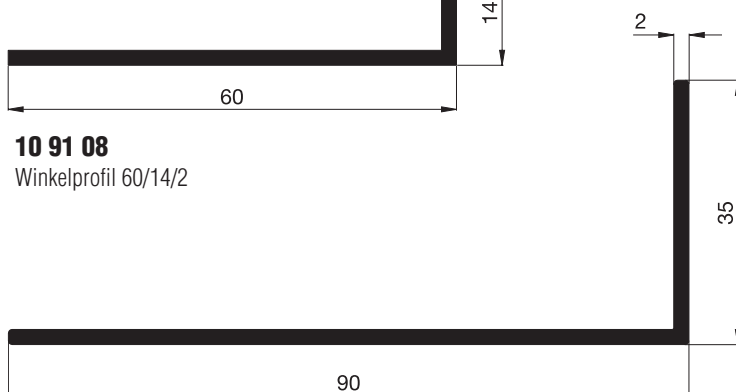
10 91 30 (nur in roh und E1 lieferbar) Winkelprofil 90/35/2
