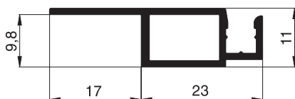
10 23 09 Spannrahmenprofil
