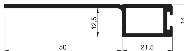
10 34 30 Montagerahmenprofil
