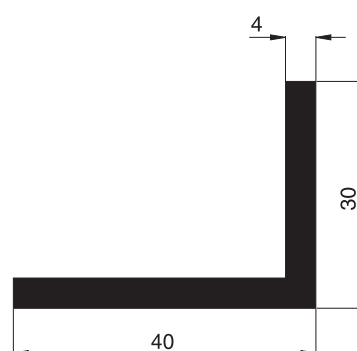
10 90 90 (nur in roh lieferbar) Winkelprofil 40/30/4
