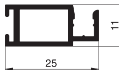
10 23 06 Spannrahmenprofil
