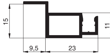
10 23 03 Spannrahmenprofil
