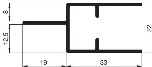
10 45 06 Rahmenprofil
