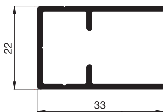
10 45 04 Rahmenprofil
