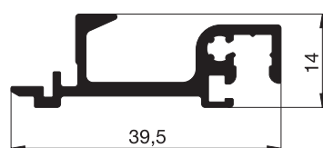
10 34 50 Griffleistenprofil
