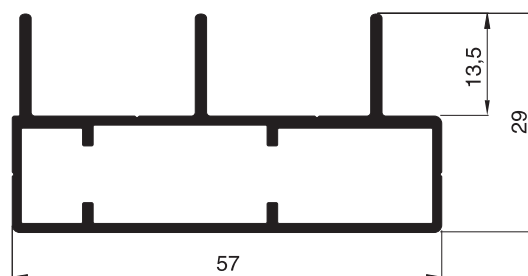
10 49 31 Laufschiene 3-fach seitlich / oben / unten
