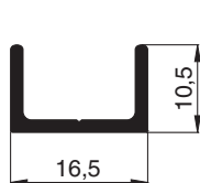
10 48 19 (nur in E1 lieferbar) Laufschiene 2-fach unten flach
