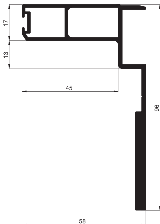
10 32 18 Statikprofil
