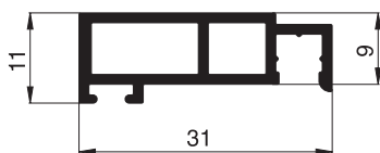
10 24 02 Spannrahmenprofil
