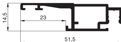
10 36 04 Drehrahmenprofil
