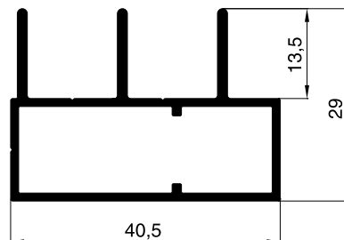
10 48 31 Laufschiene 3-fach seitlich / oben / unten
