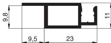
10 23 05 Spannrahmenprofil
