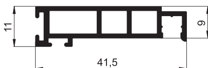
10 24 56 Spannrahmenprofil
