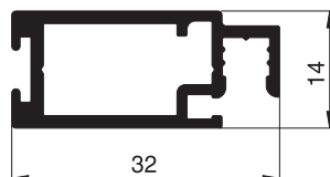
10 34 06 Pendeltürprofil
