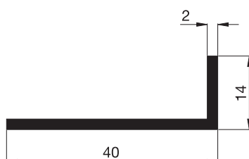
10 90 78 Winkelprofil 40/14/2
