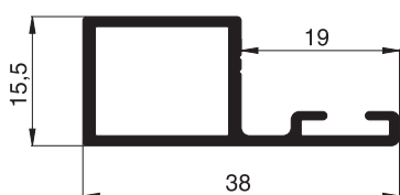
10 35 21 Montagerahmenprofil
