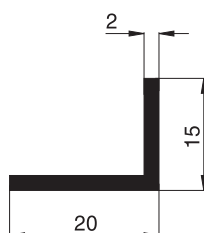
10 90 40 Winkelprofil 20/15/2
