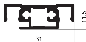
10 36 11 Sprossenprofil
