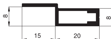
10 23 13 Montagerahmenprofil
