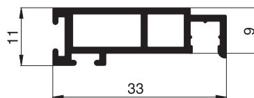
10 24 06 Spannrahmenprofil
